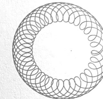
SATURN - PLUTO
