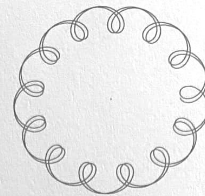
JUPITER - NEPTUNE
