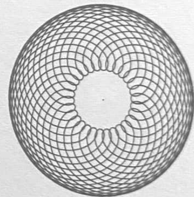
CERES - JUPITER
