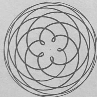
VENUS - EARTH
