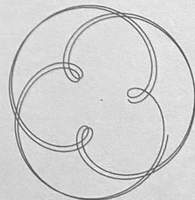
JUPITER - SATURN
