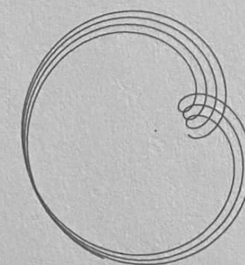
URANUS - NEPTUNE
