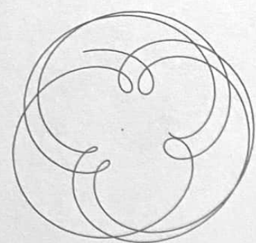
MERCURY - VENUS
