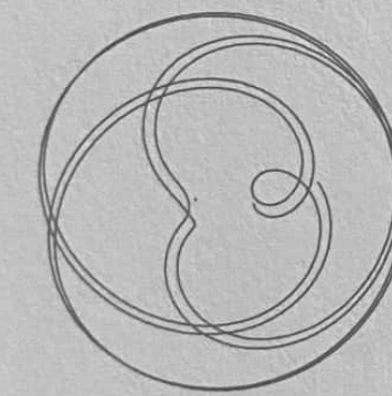
CHIRON - URANUS
