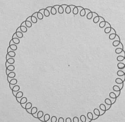
VENUS - SATURN
