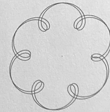
JUPITER - URANUS
