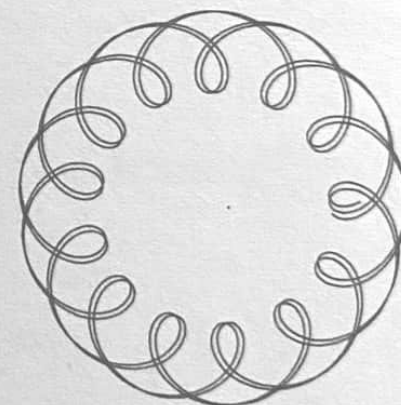
VENUS - CERES
