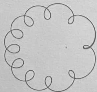
CERES - CHIRON
