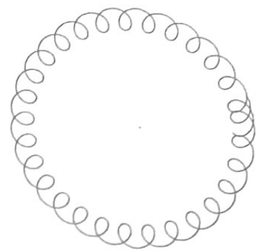
EARTH - SATURN
