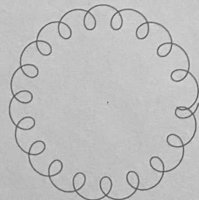
VENUS - JUPITER
