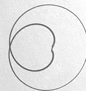
NEPTUNE - PLUTO
