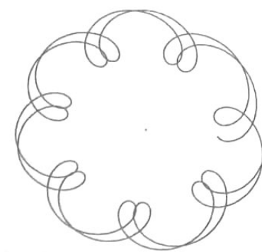
MERCURY - MARS
