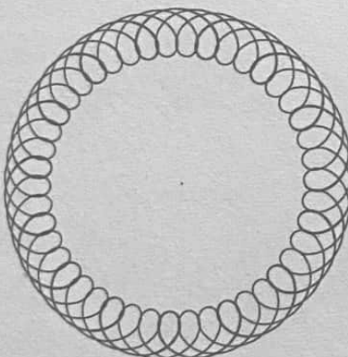
MARS - SATURN
