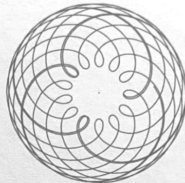
MARS - CERES
