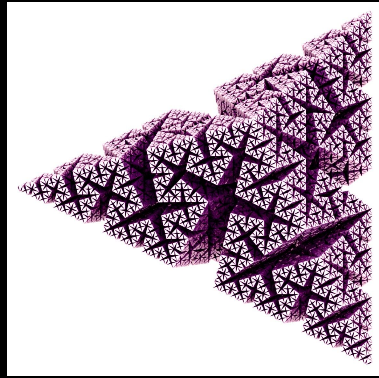
Koch bock
