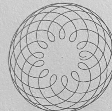
SATURN - URANUS
