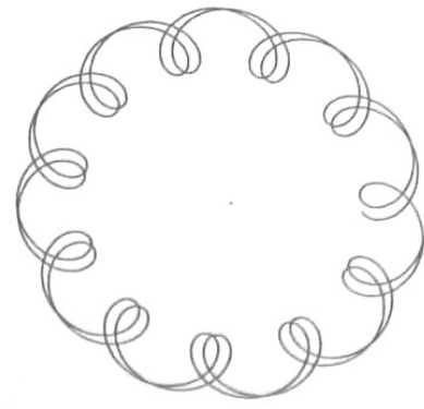
EARTH - JUPITER
