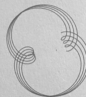
URANUS - PLUTO
