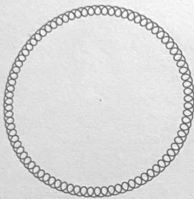
EARTH - URANUS
