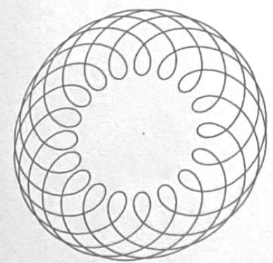
EARTH - CERES
