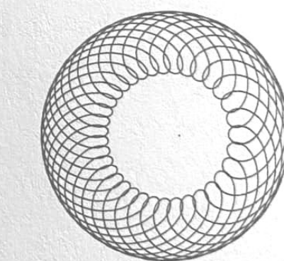
CHIRON - PLUTO
