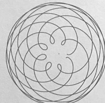
EARTH - MARS
