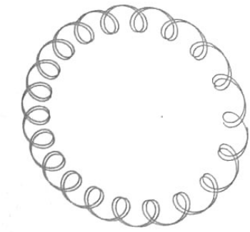
JUPITER - PLUTO
