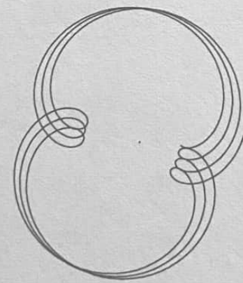
VENUS - MARS
