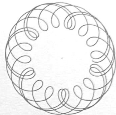
MARS - JUPITER
